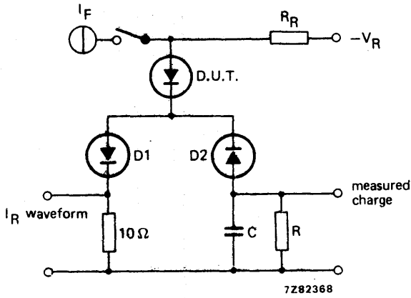
Fig. 2 Test circuit.
