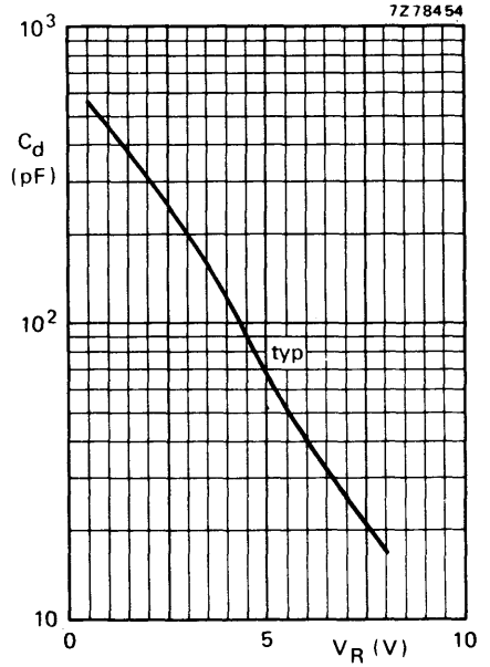
Fig. 4 f = 1 MHz.
