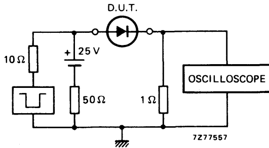
Fig. 3 Test circuit.
